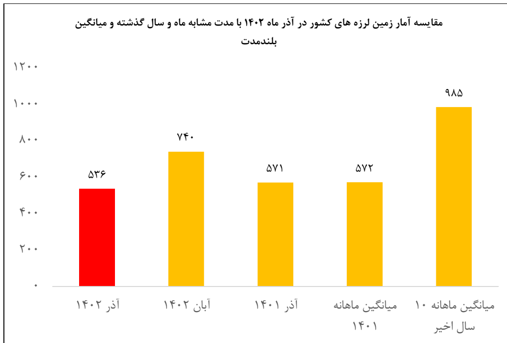
شکل ۴. آمار زمین لرزه های کشور در آذرماه ۱۴۰۲ در مقایسه با مدت مشابه سال گذشته و میانگین ماهانه ۱۰ سال اخیر
