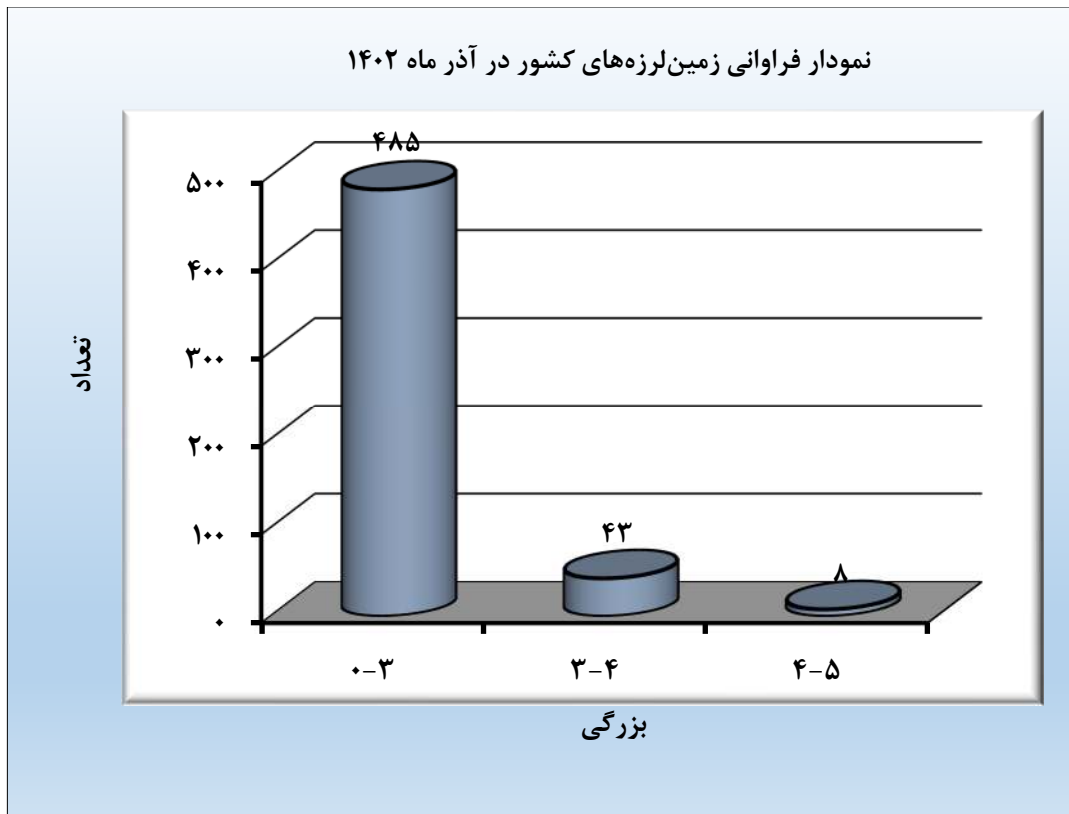
شکل ۲. نمودار میله ای فراوانی زمین‌لرزه‌های آذرماه ۱۴۰۲ به تفکیک بزرگی
