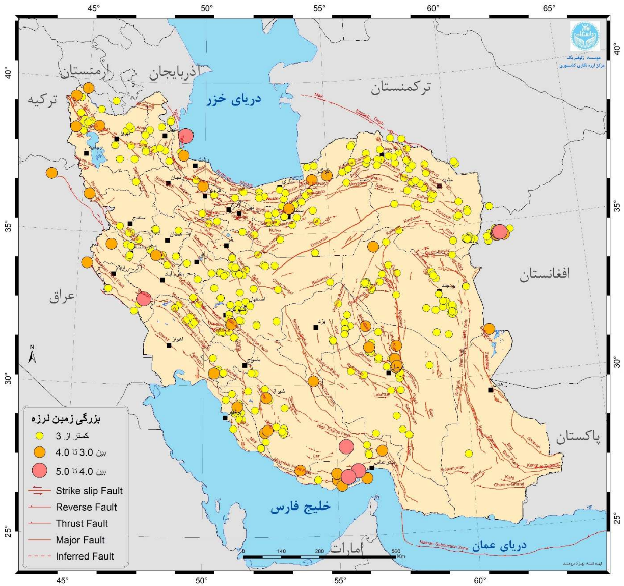
شکل ۱. نقشه پراکندگی زمین لرزه های کشور در آذرماه ۱۴۰۲
