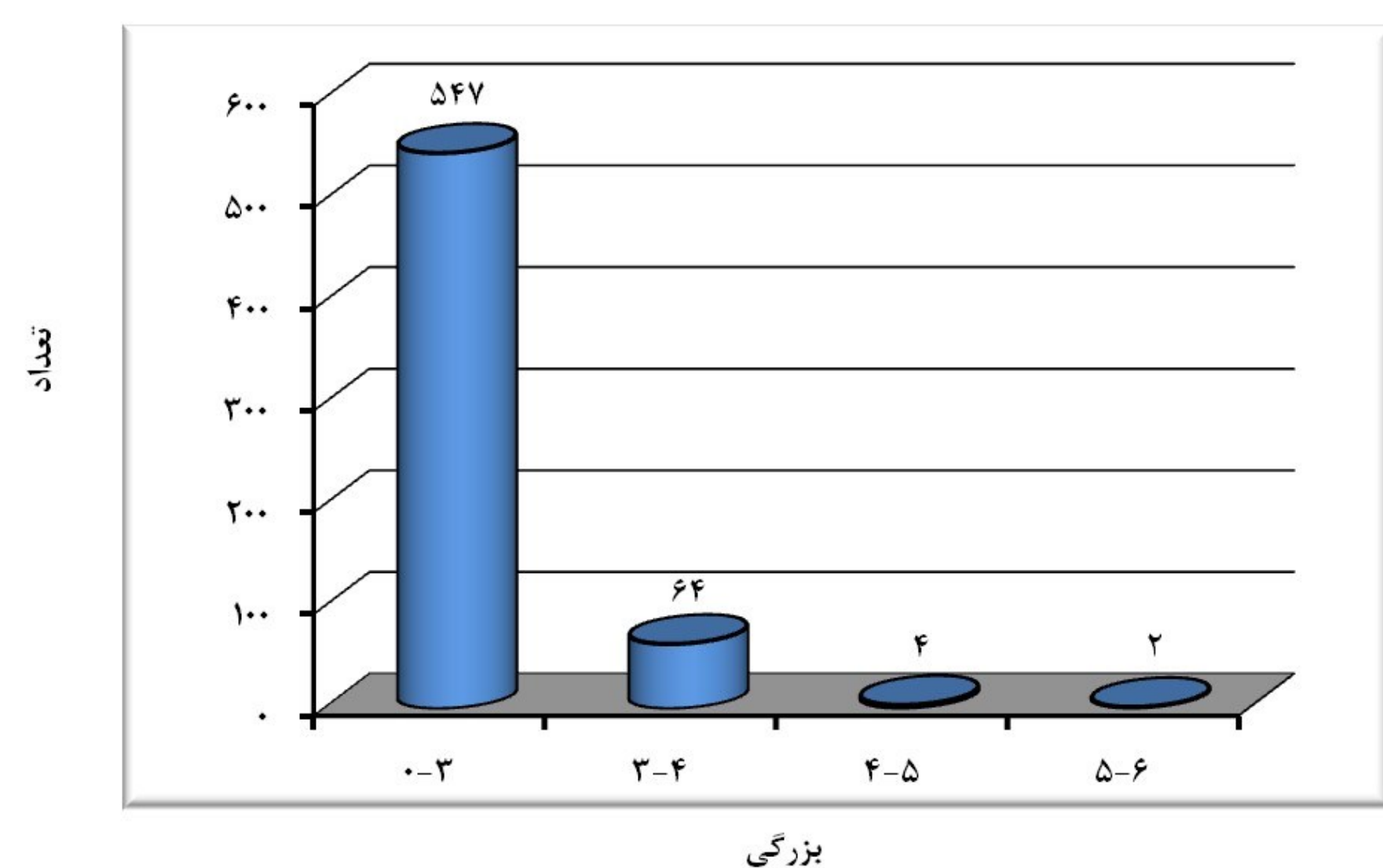
نمودار فراوانی زمین‌لرزه‌های کشور در اردیبهشت ۱۴۰۴
