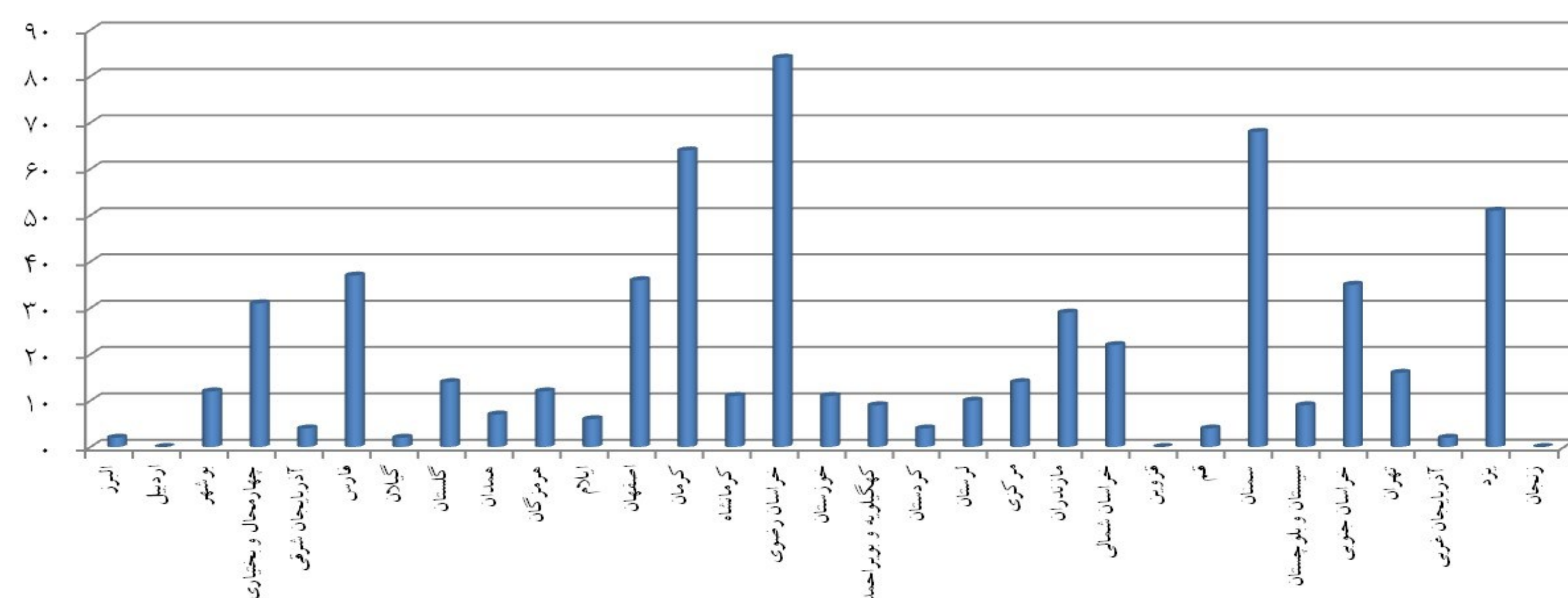
نمودار فراوانی زمین‌لرزه‌های استان‌های کشور در اردیبهشت ۱۴۰۴
